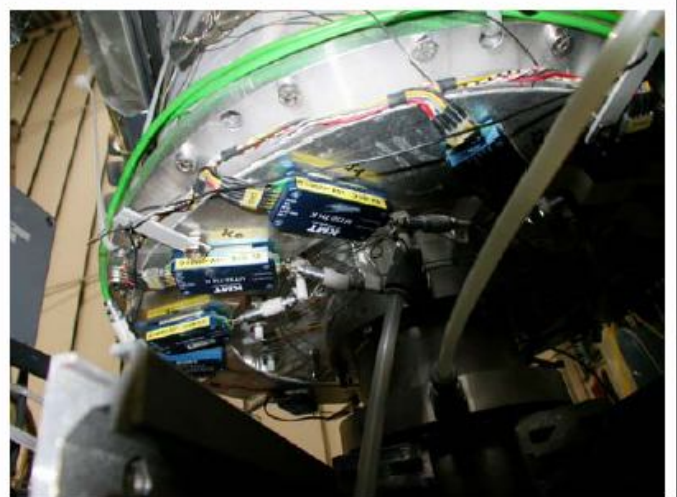
Измерения температуры вращающихся печей
